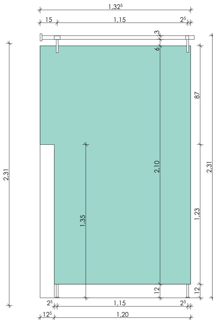
NÉZET: M=1:20
