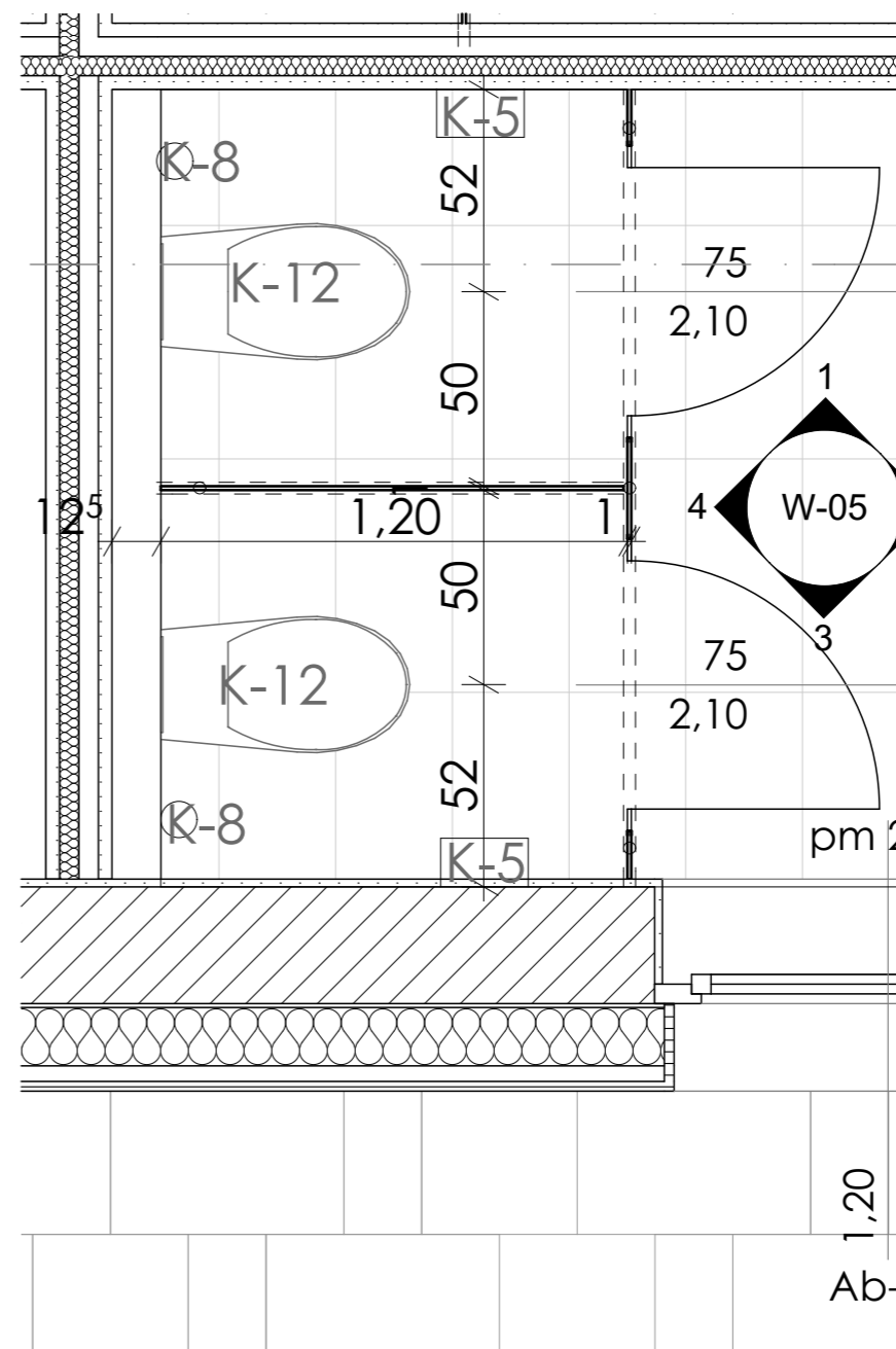
ALAPRAJZ: M=1:20
