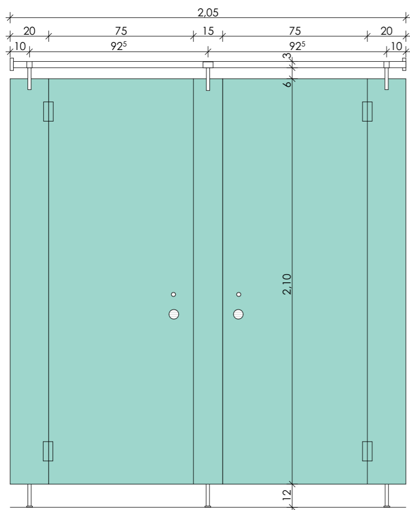
NÉZET: M=1:20
